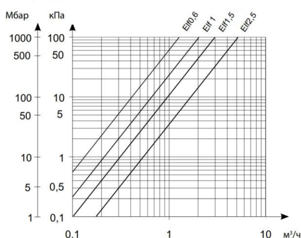
Рисунок 1. Потери давления на проточной части теплосчётчика.
