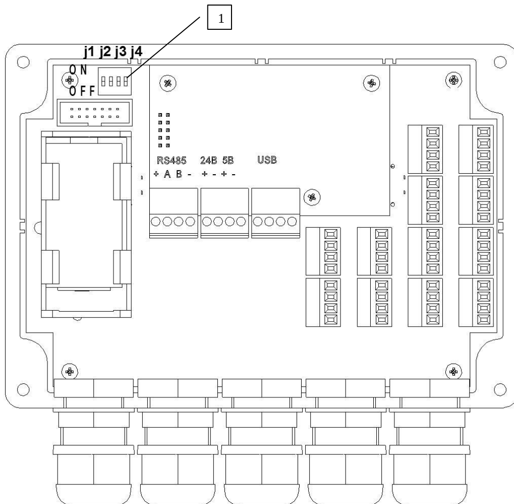
Рис.14. Расположение функциональных переключателей ВТЭ-1 (модификация СТ 10 ПМ)
