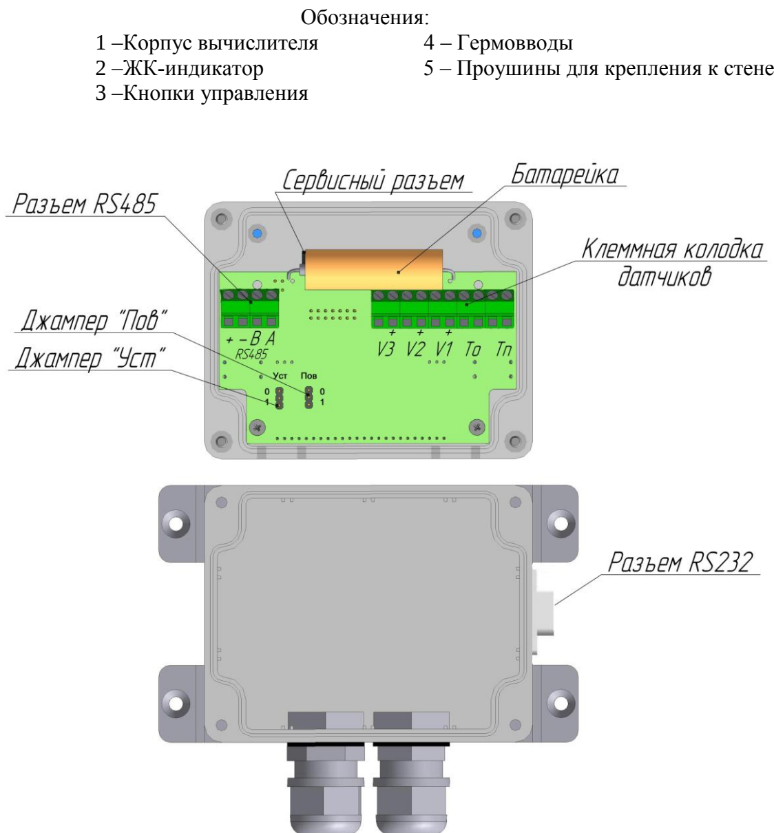
Рис.5. Конструкция тепловычислителя ВТЭ-1К-М.
