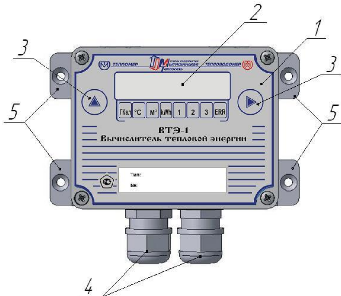
Рис.6. Внешний вид и конструкция тепловычислителя ВТЭ-1К.
