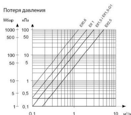
Рис.1 Потери давления на проточной части теплосчетчика.
