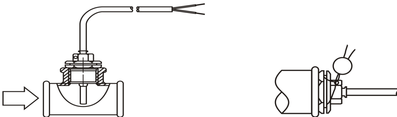
Рис. 4. Монтаж термопреобразователя сопротивления в штупцере при помощи ниппеля и пломбирование.
