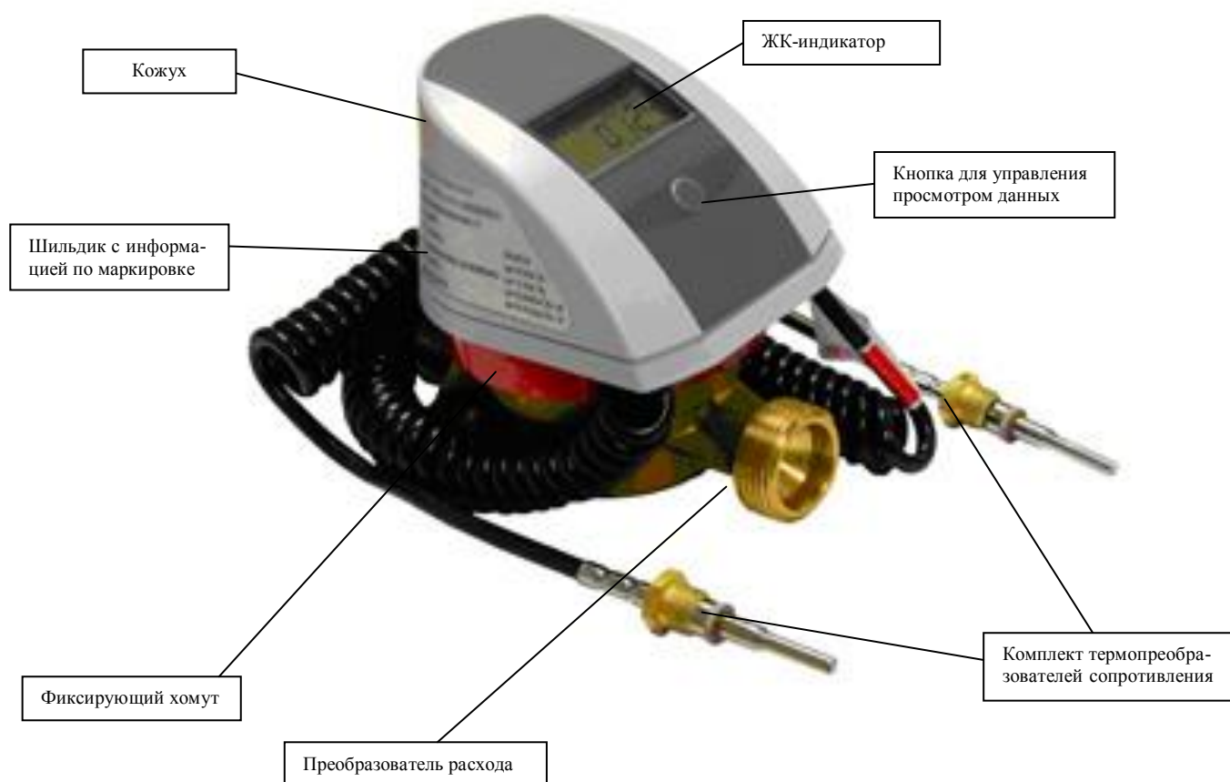
Рисунок 2. Внешний вид и состав теплосчетчика «ELF-M»
