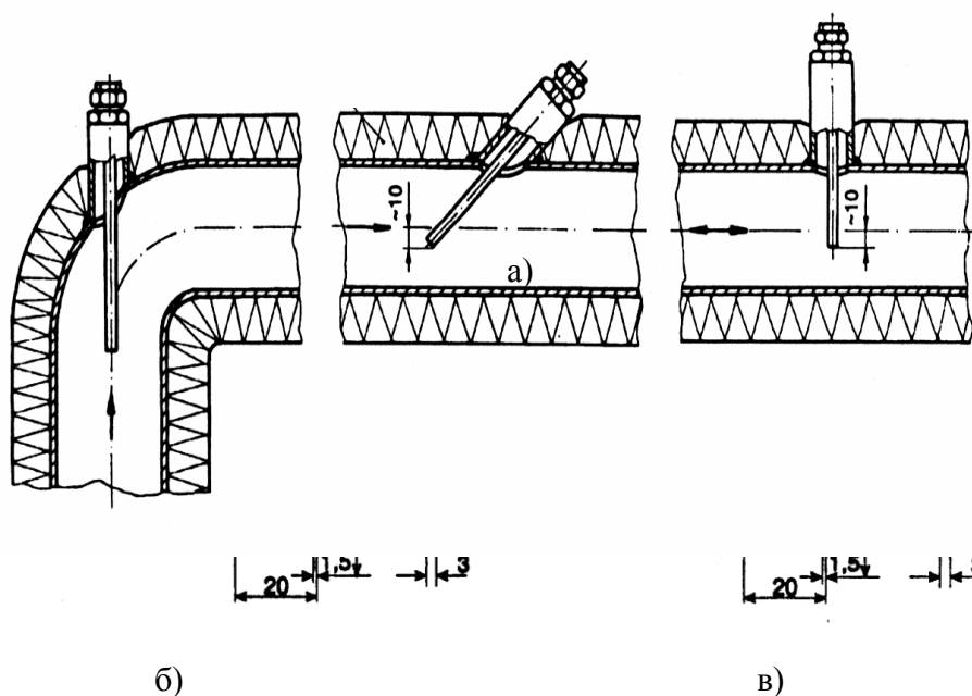
Рис. 4. Монтаж термометров сопротивления.
