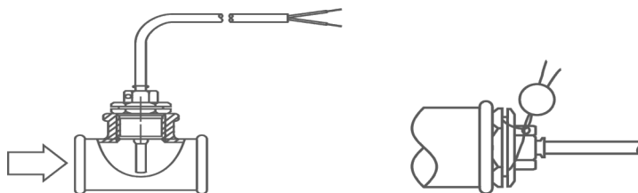
Рис.4 Монтаж и пломбирование термопреобразователя сопротивления в штупцере при помощи ниптеля.
