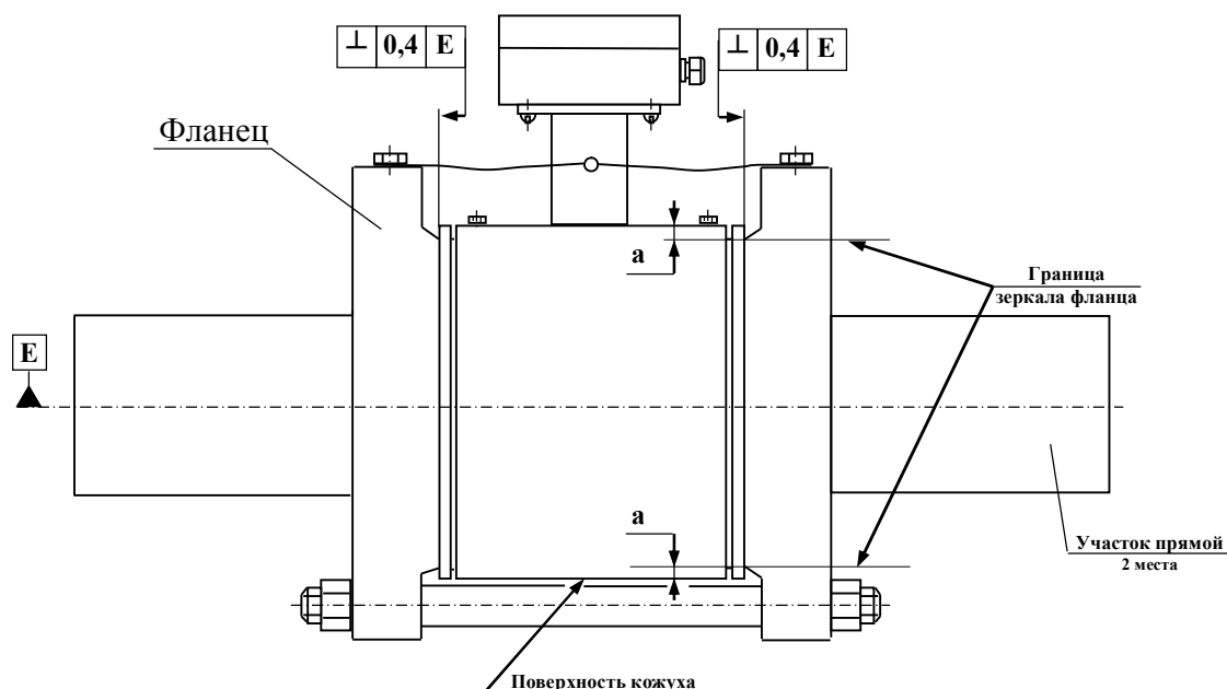
Рисунок А.9 – Требования к точности установки фланцев прямых участков
